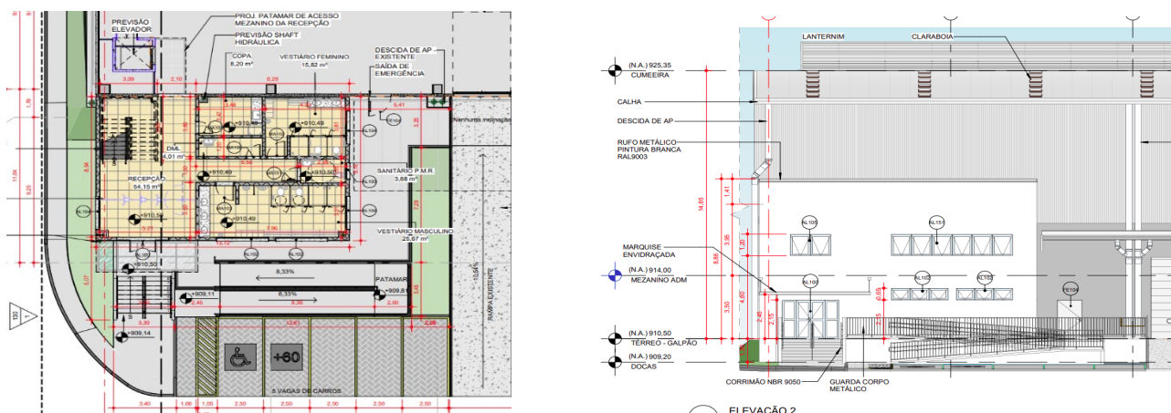
Planta piso térreo e elevação frontal da nova recepção do módulo 14.
