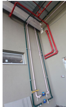
Fachada frontal; interligação das instalações de água fria, água de reuso e incêndio; finalização da interligação do esgoto.
